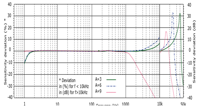
Fig 4a: Réponse en fréquence
